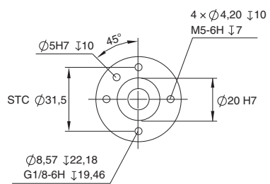
Gripper dimensions
